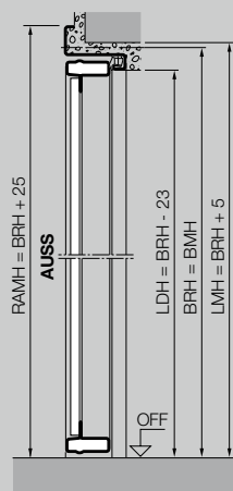
Coupe verticale – Porte sans seuil
