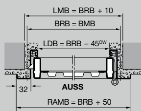
Coupe horizontale
