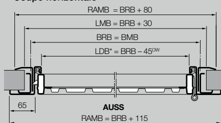
Coupe horizontale
