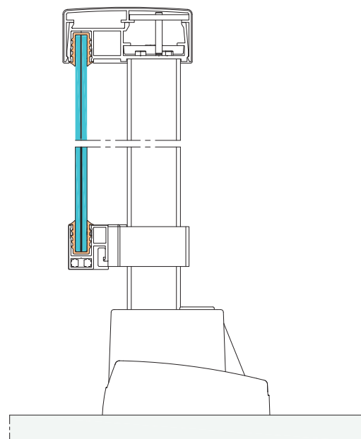
Coupe verticale
