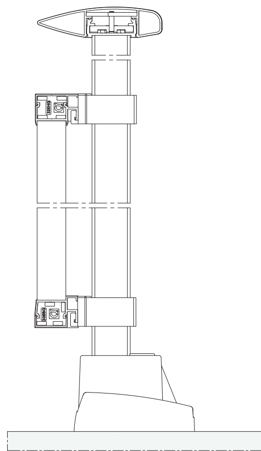
Coupe verticale
